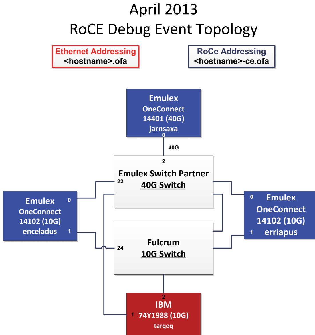
Figure 3 RoCE Interop Setup
